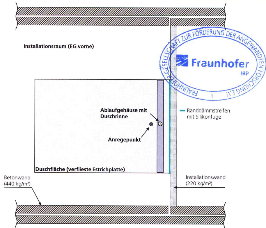
Lage des Prüfaufbaus im Installationsraum (EG vorne).
